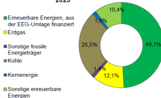
Gesamtenergieträgermix Deutschland 2023
